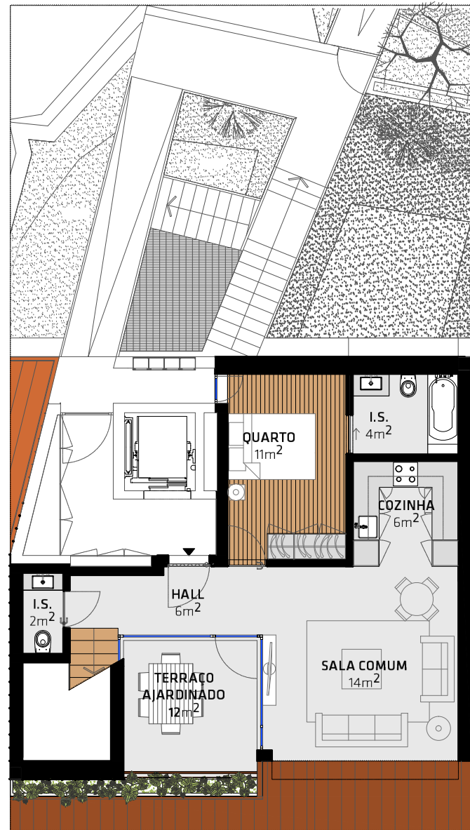
PISO 4
