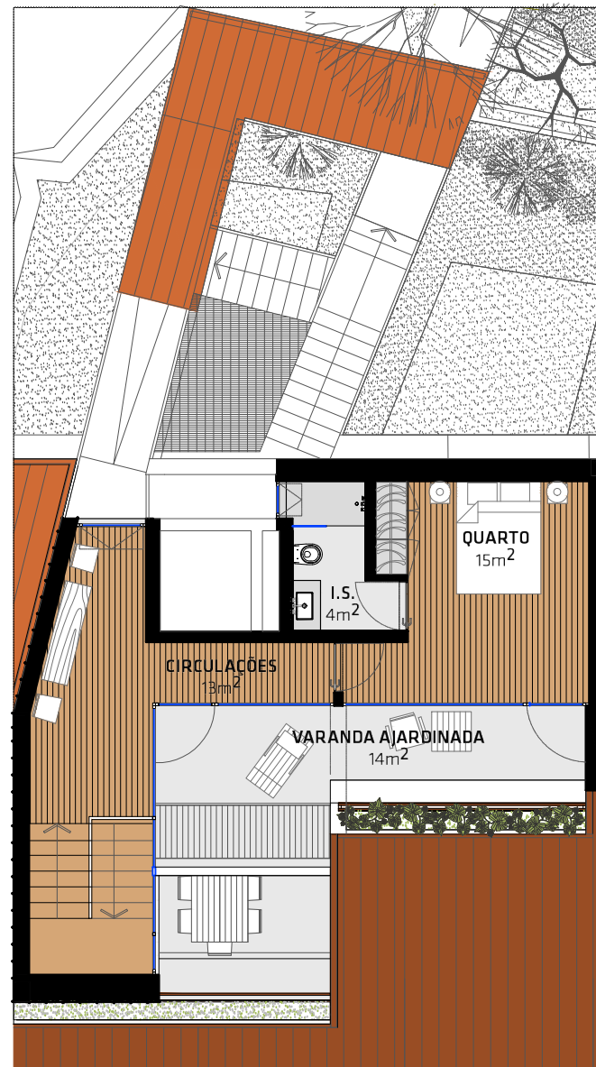
PISO 5
